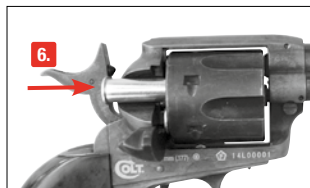
6. Coloque los cartuchos en el tambor.
