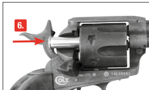
6. Patronen in die Trommel einsetzen.
